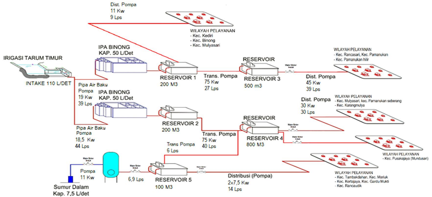
SKEMATIK SPAM PAMANUKAN DAN BINONG
