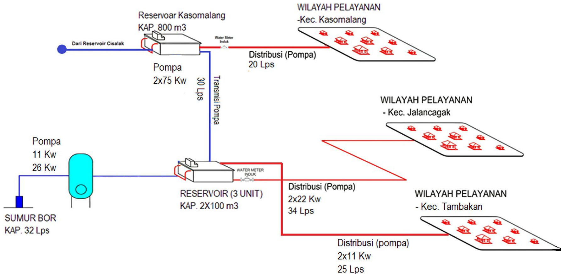
SKEMATIK SPAM JALANCAGAK
