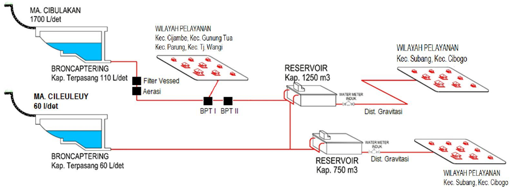
SKEMATIK SPAM SUBANG
