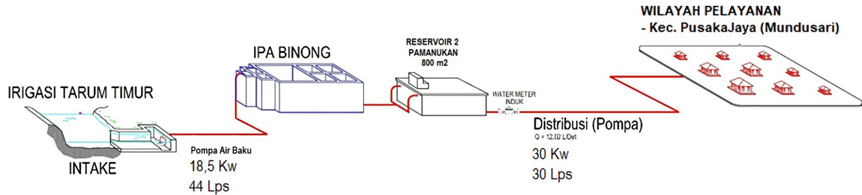
SKEMATIK SPAM PUSAKAJAYA
