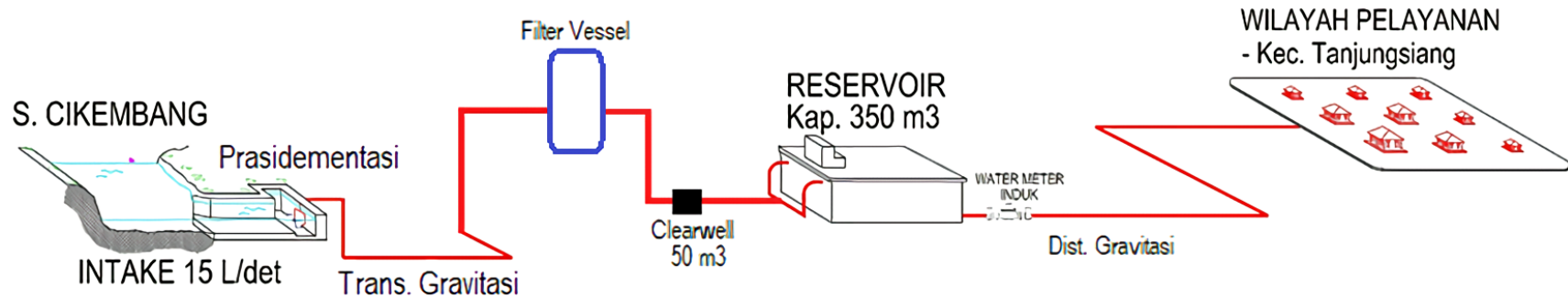
SKEMATIK SPAM TANJUNGSANG
