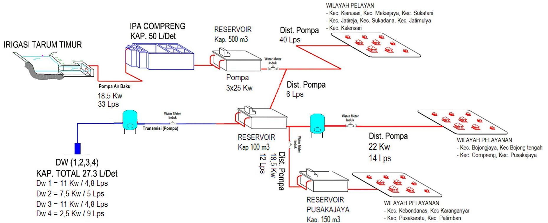
SKEMATIK SPAM COMPRENG
