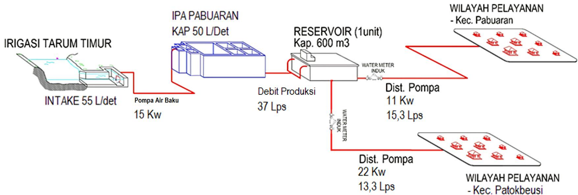
SKEMATIK SPAM PABUARAN
