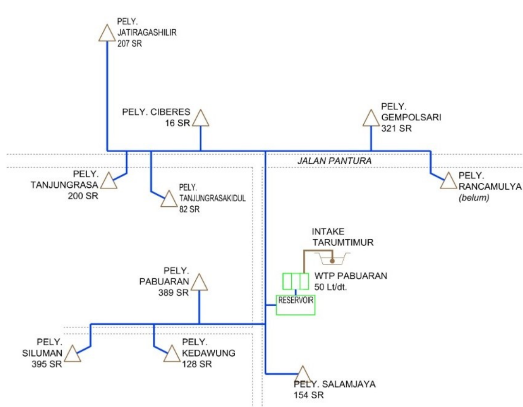
SKEMATIK SISTEM SPAM PABUARAN
