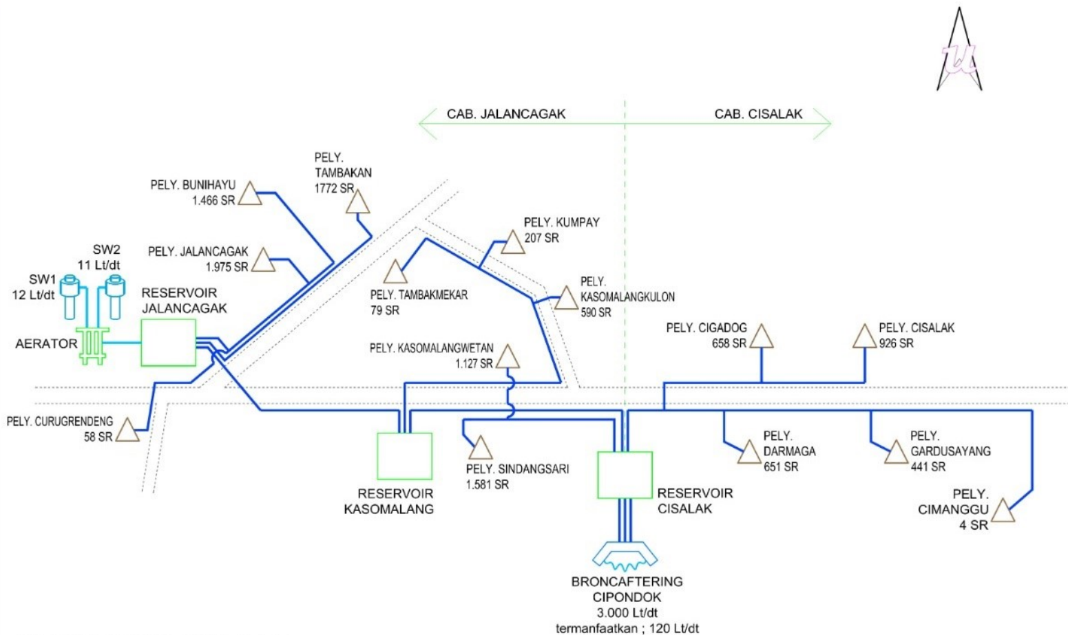
SKEMATIK SISTEM SPAM JALANCAGAK & CISLAK
